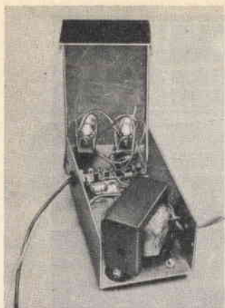
Fig. 3 - Lasciate spazio sufficiente affinché le ghiera delle lampadine restino opportunamente distanziate dalla basetta d'ancoraggio quando si fissano insieme le due metà della scatola. Le lampadine al neon possono essere montate mediante gommini o con portalamпада.
