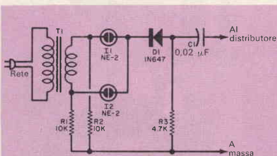
Fig. 2 - Gli impulsi provenienti dalla bobina di accensione dell'auto vengono scanditi dai 50 Hz della rete e fanno emettere dalle due lampadine al neon (I1 e I2) un segnale di calibratura.
