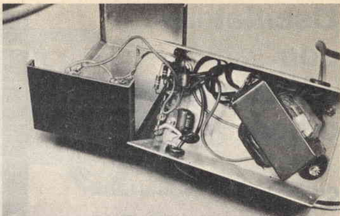
Fig. 3 - Lasciate spazio sufficiente affinché le ghiera delle lampadine restino opportunamente distanziate dalla basetta d'ancoraggio quando si fissano insieme le due metà della scatola. Le lampadine al neon possono essere montate mediante gommini o con portalamпада.
