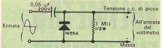
Sonda rivelatrice per la misura di basse tensioni di picco c.a. Per il filtraggio è sufficiente la capacità tra i fili della sonda stessa.
